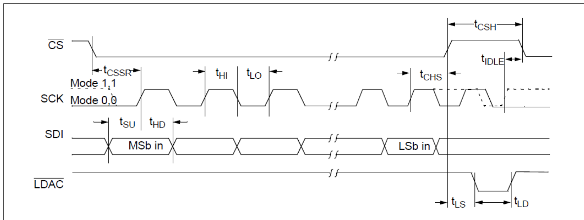
FIGURE 1-1: SPI Input Timing Data.
